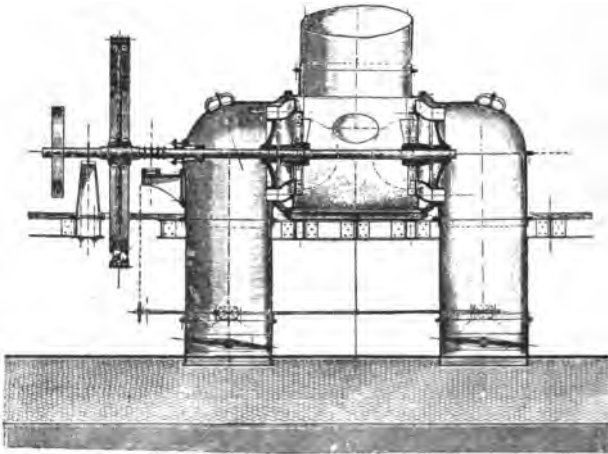
Fig. 49. Penstock-Jonval-Turbine der Maschinenfabrik Oerlinggen.
